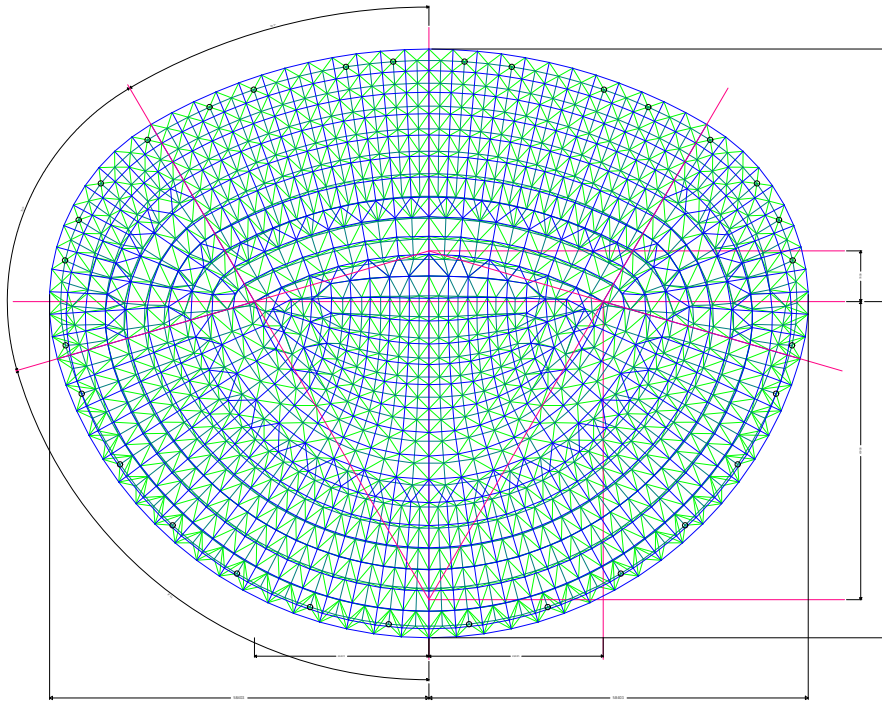
GENERAL LAY-OUT
