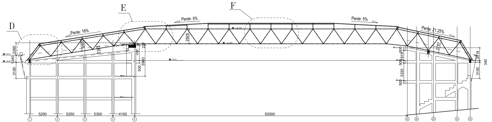
Coupe Longitudinale
