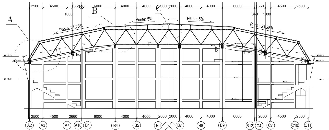
Coupe Transversale
